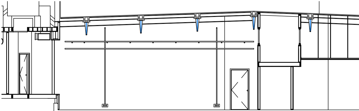
Longitudinal Section
